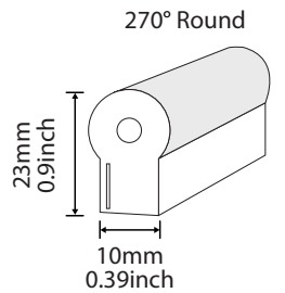
D1023 Profile
